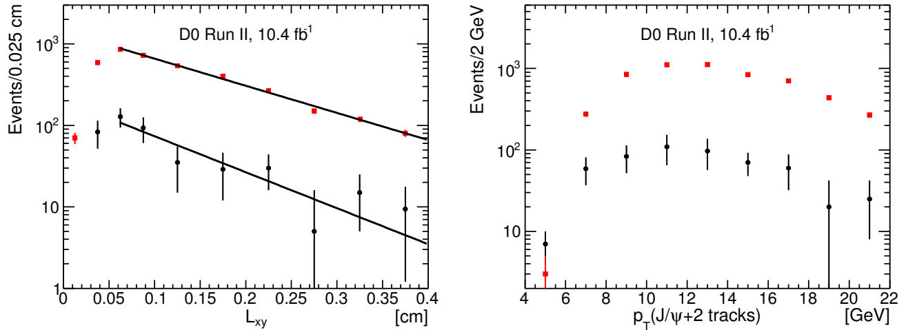
Рисунок 4.7 — Слева: Распределение по L_{xy} для событий Z_c^\pm(3900) (черные кружки) и B_d^0 \rightarrow J/\psi K^* (красные квадраты). Справа: Распределение по p_T системы J/\psi \pi^+ \pi^- , являющейся “родительской” для Z_c^\pm(3900) (черные кружки) и B_d^0 \rightarrow J/\psi K^* (красные квадраты).
