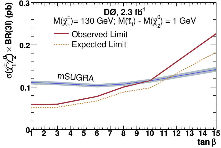
Рисунок 2.10 — Верхний предел по уровню значимости 95% на \sigma \times \text{BR}(3l) в зависимости от \tan \beta , в сравнении с предсказанием модели mSUGRA для массы чаржино 130 ГэВ/ c^2 и m_{\tilde{\tau}} - m_{\tilde{\chi}_2^0} = 1 ГэВ/ c^2 .
