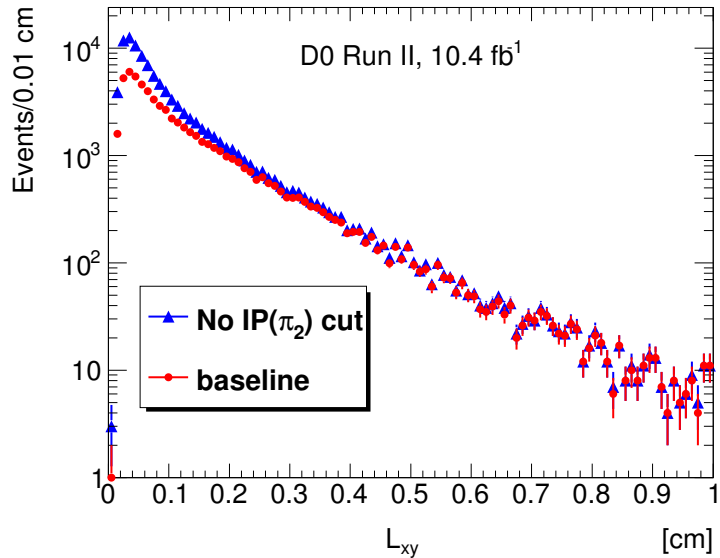
Рисунок 4.3 — Распределение по поперечной длине распада L_{xy} для отобранных кандидатов J/\psi\pi^+\pi^- в диапазоне инвариантных масс 4.2 < M(J/\psi\pi^+\pi^-) < 4.7 \text{ ГэВ}/c^2 (красные кружки). Также показано подобное распределение, но без применения условия на значимость прицельного параметра второго пиона (синие треугольники).
