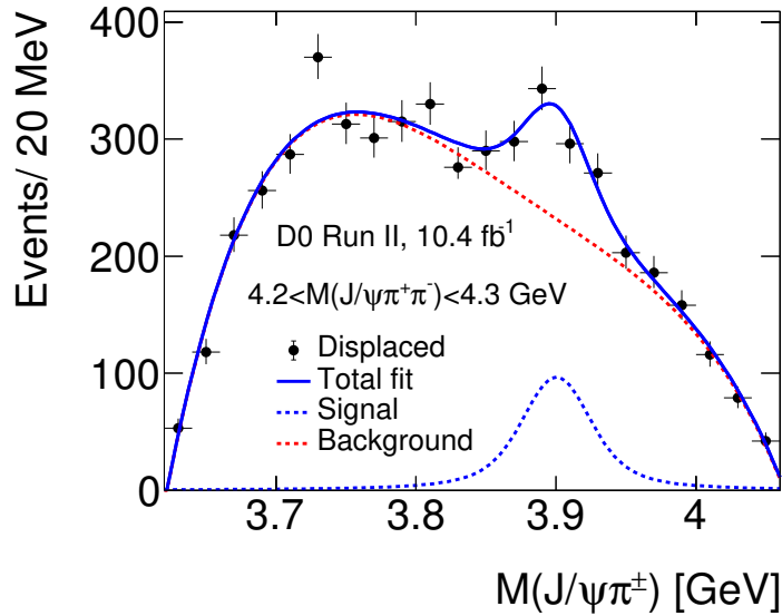
Рисунок 4.13 — Распределение по инвариантной массе M(J/\psi\pi^\pm) для событий в диапазоне 4.2 < M(J/\psi\pi^+\pi^-) < 4.3 \text{ ГэВ}/c^2 и набора “смещенной вершины”. Сплошной линией показан общий результат фита; синей штриховой линией показан сигнал, параметризованный с помощью функции релятивистского Брейт-Вигнера с нефиксированной массой и шириной; красной штриховой линией показан фон, параметризованный с помощью полиномов Чебышева четвертого порядка.
