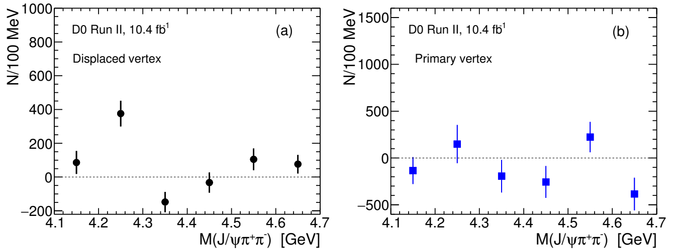
Рисунок 4.12 — Выходы сигнала Z_c^\pm(3900) на бин шириной 100 МэВ для шести интервалов по M(J/\psi\pi^+\pi^-) : 4.1–4.2, 4.2–4.3, 4.3–4.4, 4.4–4.5, 4.5–4.6 и 4.6–4.7 \text{ГэВ}/c^2 для (а) набора “смещенной вершины” и (б) набора “первичной вершины”. Точки располагаются в центрах соотв. бинов.
