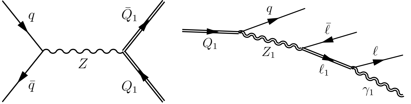
Рисунок 2.11 — Диаграмма, представляющая парное рождение KK -кварков ( Q_1 ) — слева, с последующим каскадным распадом Q_1 на KK -состояния, соответствующие калибровочному бозону ( Z_1 ), лептону ( l_1 ) и фотону ( \gamma_1 ) плюс частицы стандартной модели (кварки и лептоны) — справа.
