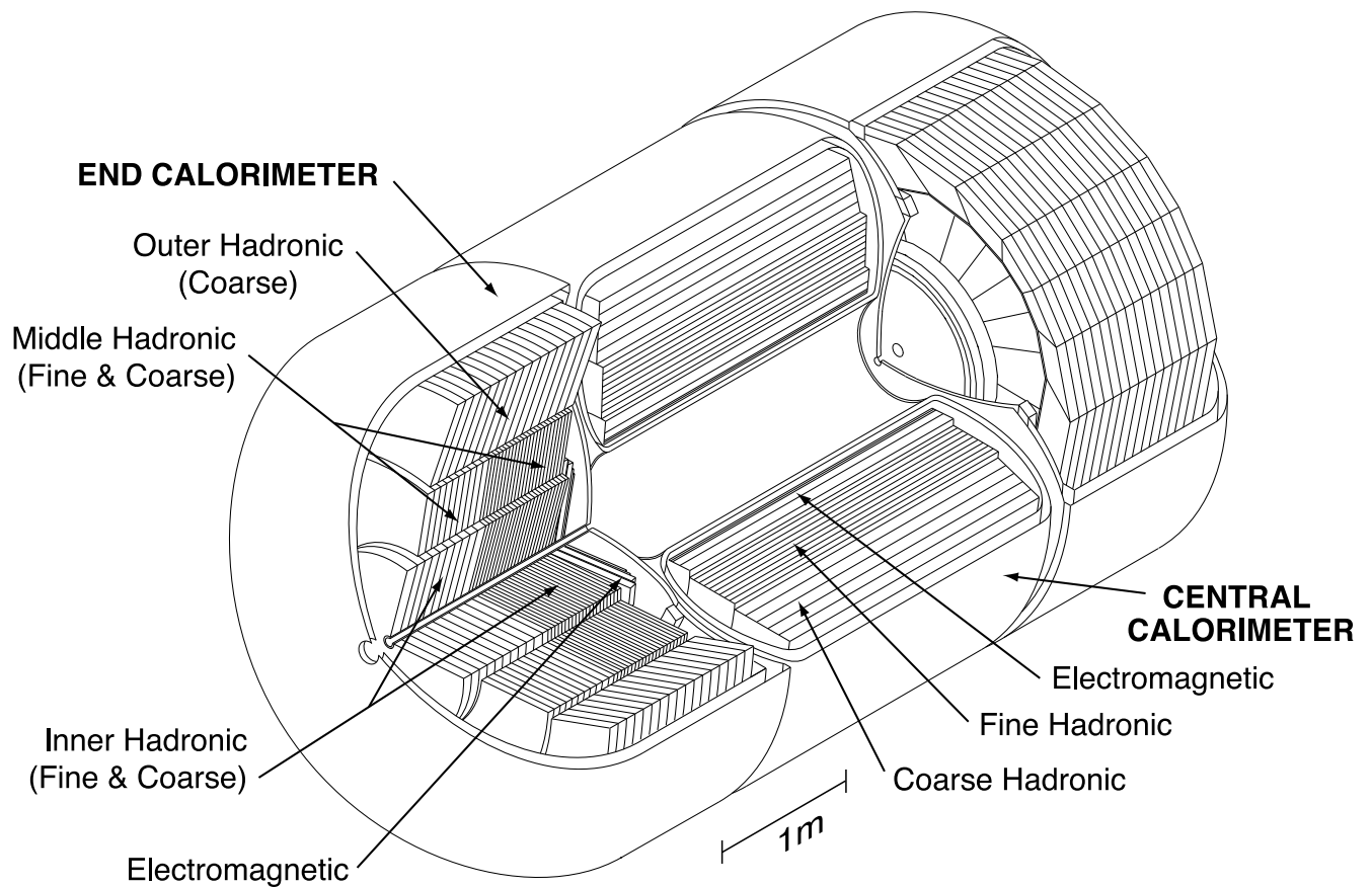
Рисунок 1.3 — Общий вид на центральный и два торцевых калориметра в изометрической проекции.
