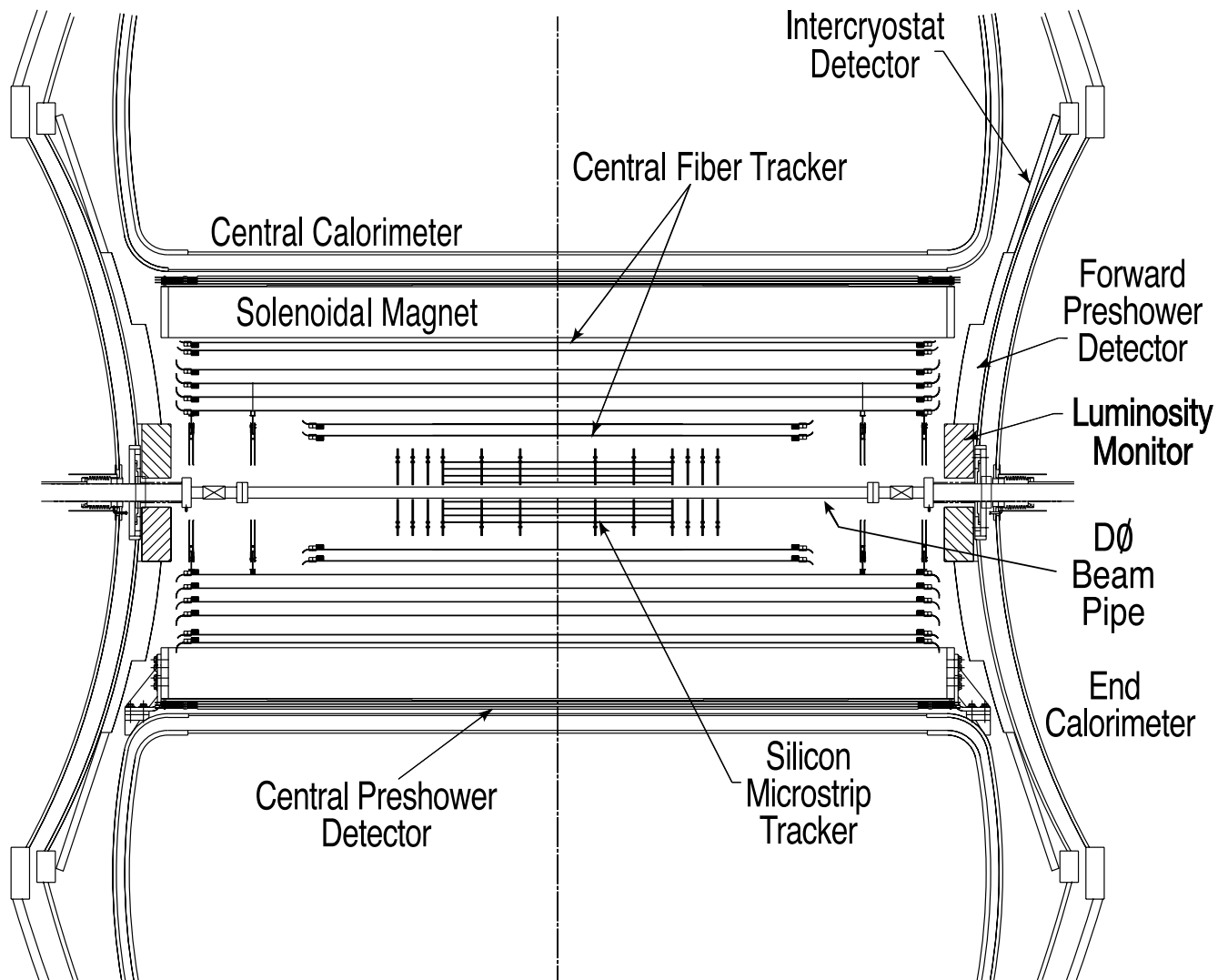
Рисунок 1.2 — Вид в разрезе на центральную трековую систему. Также показаны соленоид, предливневые детекторы, монитор светимости и калориметрическая система.
