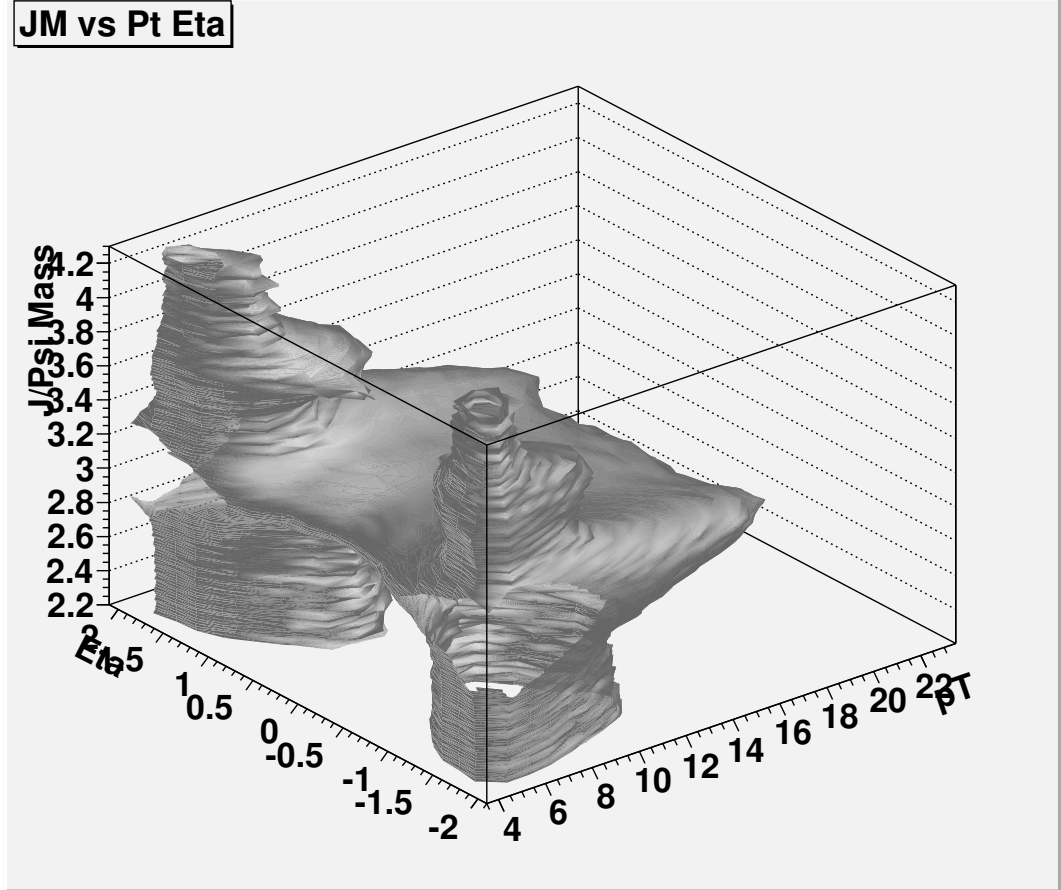
Рисунок 3.14 — “Изотермическая” поверхность 3-D распределения H(M_{\mu\mu}, p_T^{J/\psi}, \eta^{J/\psi}) для отобранных кандидатов в SJ события (детали в тексте).
