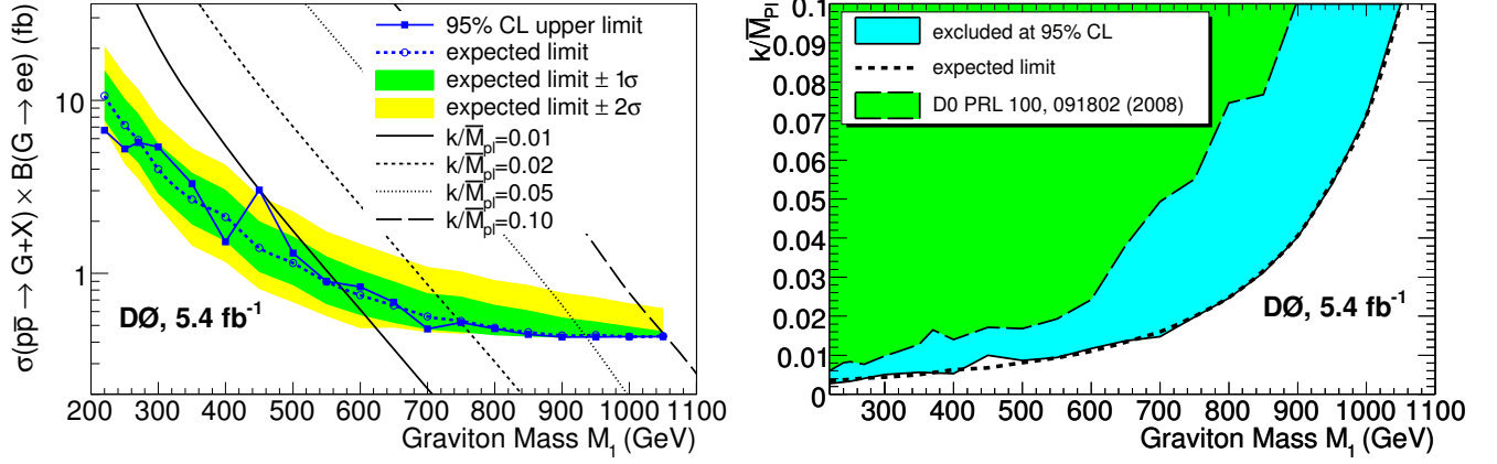
Рисунок 2.13 — Слева: верхний предел на сечение \sigma(p\bar{p} \rightarrow G + X) \times Br(G \rightarrow ee) по уровню значимости 95% в сравнении с ожидаемым пределом и теоретическими предсказаниями для различных значений параметра k/\bar{M}_P . Справа: верхний предел на k/\bar{M}_P в зависимости от M_1 по уровню значимости 95% в сравнении с ожидаемым пределом и результатом, полученным в предыдущем анализе [28].
