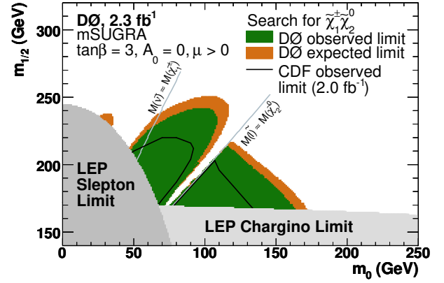
Рисунок 2.9 — Область на плоскости параметров m_0 - m_{1/2} исключенная благодаря данному анализу (зеленый цвет), поисков чаржино (слабый серый цвет) и слептонов (густой серый цвет) на LEP [19] и в эксперименте CDF (черная линия) [20]. Прочие параметры mSUGRA брались равными \tan\beta = 3, A_0 = 0, \mu > 0 .
