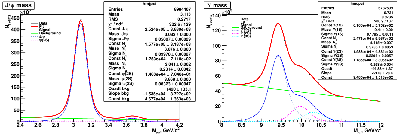
Рисунок 3.21 — Распределения по инвариантной массе двух мюонов M_{\mu\mu} для событий-кандидатов в случае одиночного рождения J/\psi (слева) и \Upsilon (справа). Красная линия - общий результат фита, синяя линия - результат для сигнала, зеленая линия - результат для фона. Пунктирные линии - индивидуальные вклады от резонансов J/\psi , \psi(2S) , \Upsilon(1S) , \Upsilon(2S) и \Upsilon(3S) .
