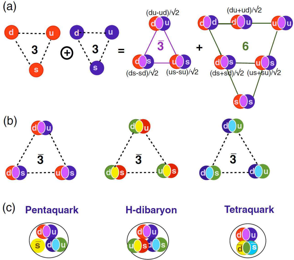
Рисунок 4.1 — (a) Комбинация красного и синего триплетов кварков приводит к пурпурным (анти-зеленым) антитриплету и секстету. Антитриплет антисимметричен и по цвету, и по аромату, секстет симметричен по аромату и антисимметричен по цвету. (b) Три антицветных антитриплета дикварков. (c) Некоторые из многокварковых бесцветных состояний могут быть построены из кварков, антикварков, дикварков и диантикварков.
