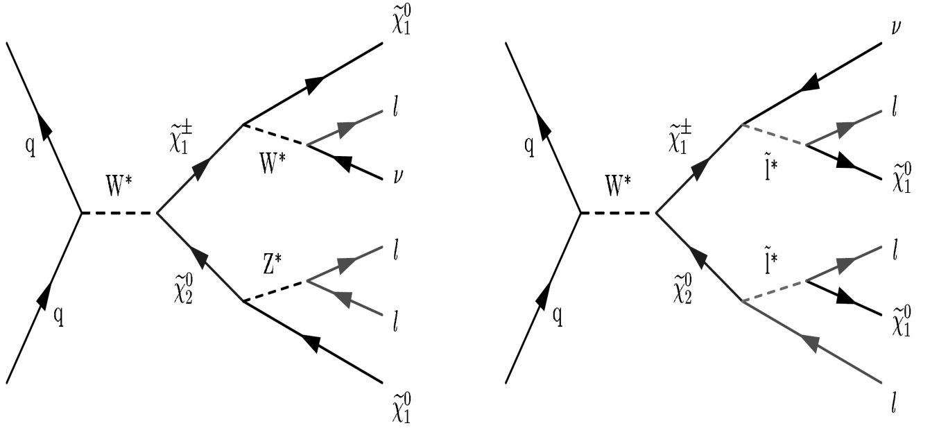
Рисунок 2.1 — Основные моды рождения и распада чаржино и нейтралино, рассматриваемые в данной работе.
