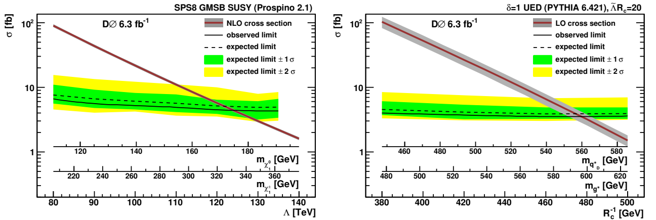
Рисунок 2.15 — Теоретические сечения для моделей GMSB (слева) и UED (справа) вместе с ожидаемыми и наблюдаемыми верхними пределами на соответствующие сечения по уровню значимости 95% в зависимости от \Lambda и R^{-1} соответственно. Для модели GMSB приведены соответствующие массы легчайших нейтралино ( \tilde{\chi}_1^0 ) и чаржино ( \tilde{\chi}_1^\pm ). Для модели UED приведены соответствующие массы КК кварка и КК глюона. Масса КК фотона приблизительно равна R^{-1} .
