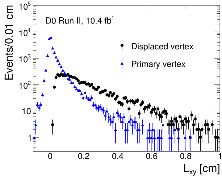
Рисунок 4.9 — Длина распада J/\psi\pi^+\pi^- в поперечной плоскости для событий в диапазоне 4.2 < M(J/\psi\pi^+\pi^-) < 4.3 ГэВ/с 2 . Черными кружками показано распределение для событий из набора “смещенной вершины”. Синими треугольниками показано распределение для событий из набора “первичной вершины” (см. текст).
