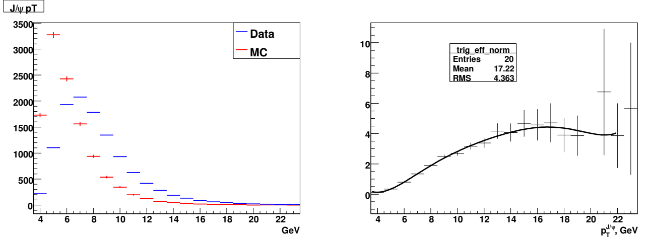
Рисунок 3.5 — Слева: Распределение по p_T(J/\psi) для данных (синие точки с ошибками) и сгенерированных событий SJ CS (красные точки с ошибками) отнормированных к данным по интегралу. Справа: Отношение данные/МС для распределений на левом рисунке с наложенным результатом фита. Подробности в тексте.
