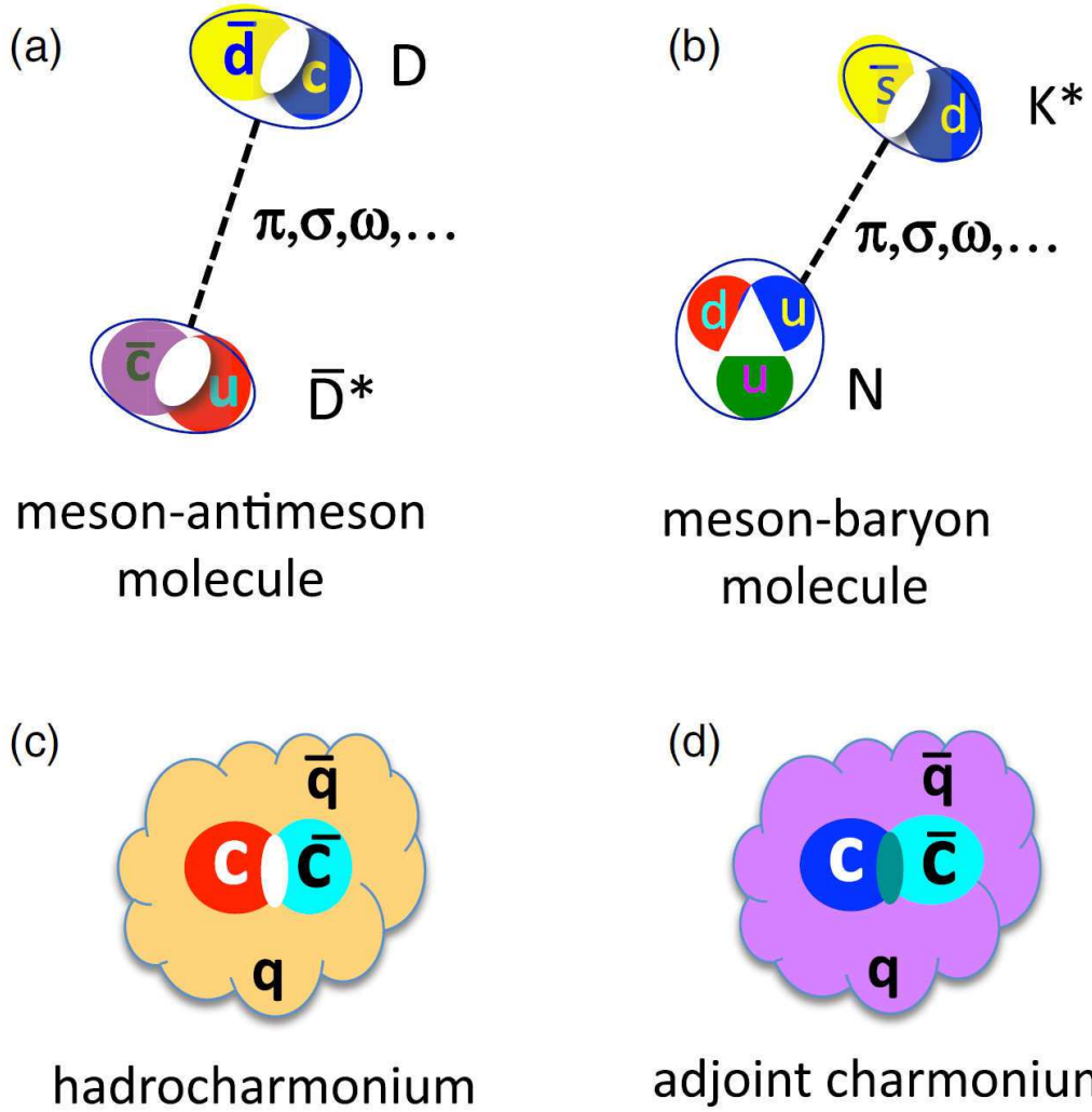
Рисунок 4.2 — (а) Мезон-мезонная и (b) мезон-барионная молекулоподобная структура, связанная взаимодействием Юкавы в форме мезонного обмена. (с) схематическое изображение структуры адрочармония, в котором бесцветное ядро из тяжелых кварков ( Q\bar{Q} ) взаимодействует с окружающей “каплей” глюонов и легких кварков с помощью КХД-версии сил Ван-дер-Ваальса. (d) Модель “присоединенного чармония”, в котором цветное Q\bar{Q} -ядро взаимодействует с окружающими глюонами и кварками через цветные силы.
