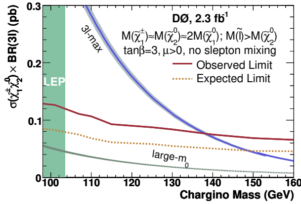
Рисунок 2.8 — Верхний предел по уровню значимости 95% на \sigma \times \text{BR}(3l) в зависимости от массы чаржино, в сравнении с ожидаемыми результатами от двух сценариев SUSY (см. текст). Ошибки рассматриваемых сценариев показаны заштрихованными полосами.
